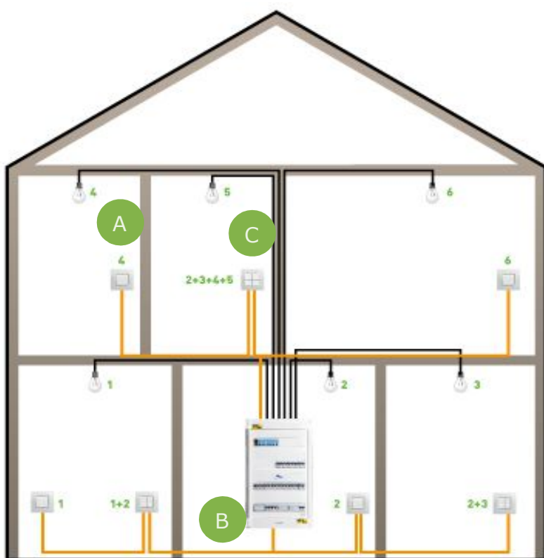
Enkelvoudige schakelaar
