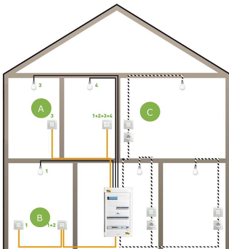
Enkelvoudige schakelaar
